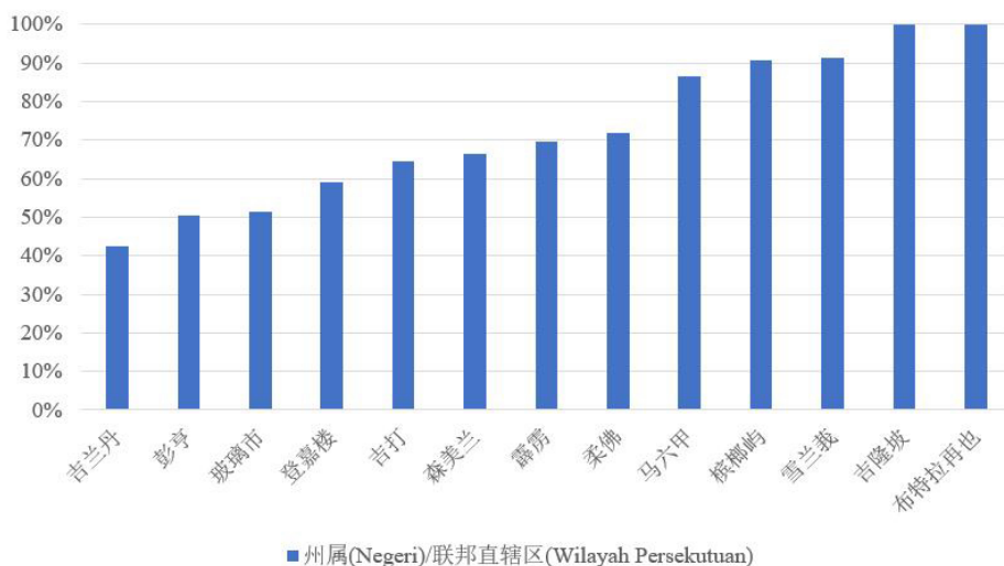
图 1 马来西亚半岛各州级行政单位城市化率(2010 年)
